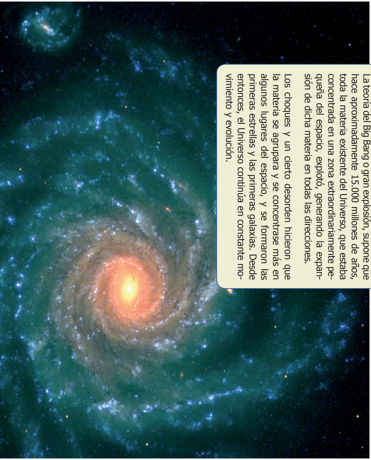
■ Galaxia Espiral NGC 1232, Foto Observatorio Europeo Austral, ESO.
